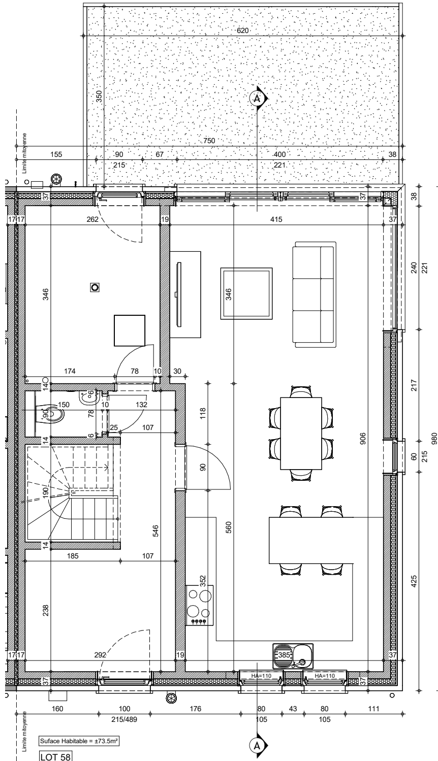
REZ-DE-CHAUSSEE
